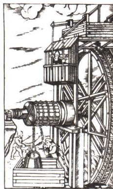
Большая водоподъемная машина. Гравюра (XVI в.).
