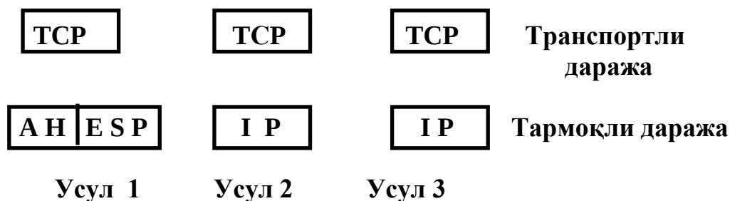
6.1-расм. Тармоқларда ахборотни ҳимоя қилишнинг учта усули
