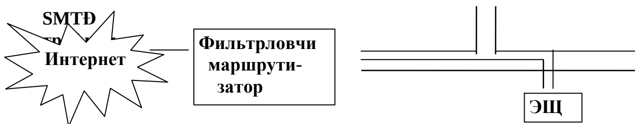
6.4-расм. SMTP ва TELNET трафикни филтрлаш схемаси
