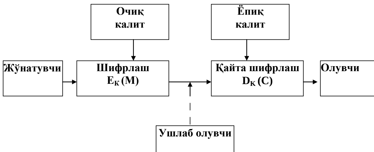
4.8- расм. Очиқ калитли носимметри криптотизимнинг умумлашган схемаси
