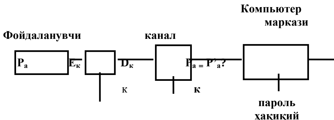
6.5-рasm. Пароль ёрдамида оддий аутентификациялаш схемаси
