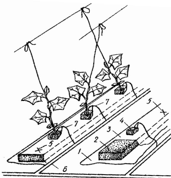
18-расм. Минерал пахтада сабзавот экинларини ўстириш принципи.
