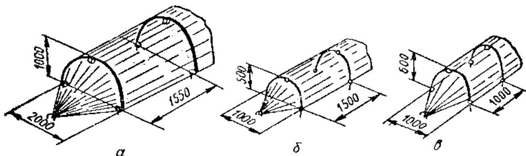
3-расм. Заводда тайёрланган тоннелли ёпқичлар: а – эгат учун; б, в – ўрқачлар учун (ўлчами мм да)
