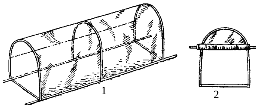
4-расм. Кичик ҳажмли плёнкали кўчма қурилма: 1 – ёнидан кўриниши; 2 – олдиан кўриниши
