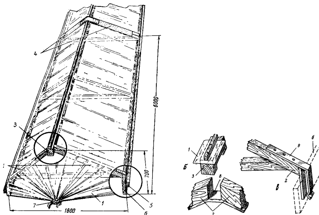
9-расм. КЙК (УРП) кўчириладиган-йиғма курилма (810-92 намунавий лойиҳа):
