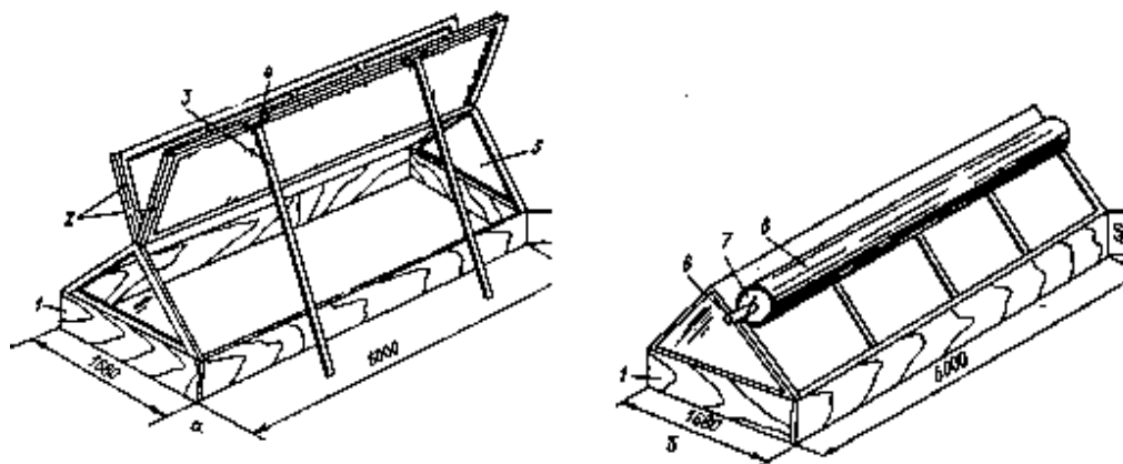
8-расм. Икки нишабли плёнкали парник.
