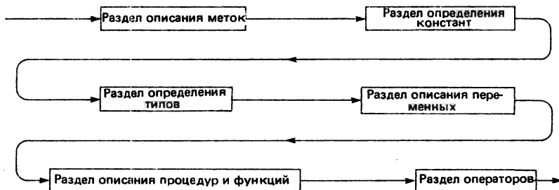
Р и с. 3.2. Синтаксическая диаграмма для Блока
