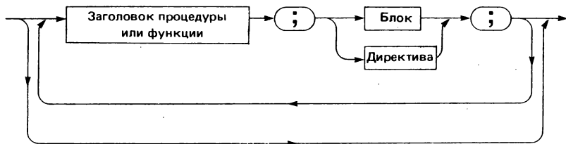
Р и с. 11.1. Синтаксическая диаграмма для Раздела описания процедур и функций
