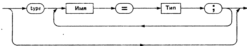
Р и с. 3.8. Синтаксическая диаграмма для Раздела определения типов
