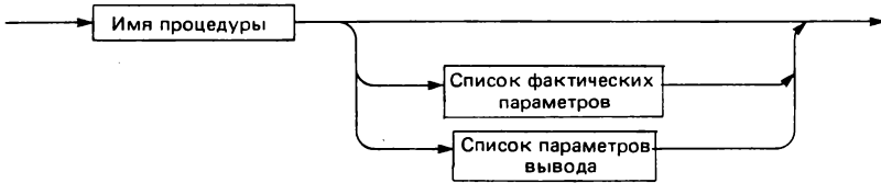
Рис. 11.4. Синтаксическая диаграмма для Оператора процедуры
