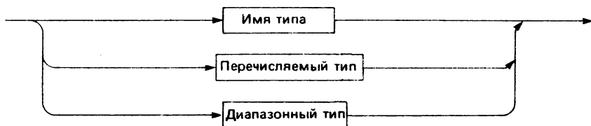
Р и с. 2.4. Синтаксическая диаграмма для Ординального типа
