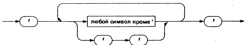
Рис. 1.6. Синтаксическая диаграмма для Строки символов
