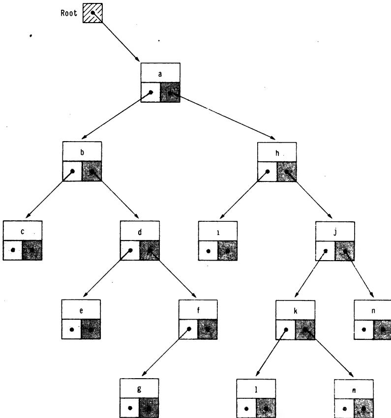
Р и с. 11.9. Стрoение двоичного дерева
