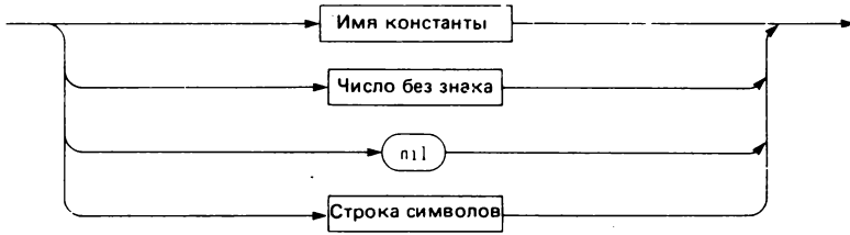
Рис. 4.5. Синтаксическая диаграмма для Константы без знака
