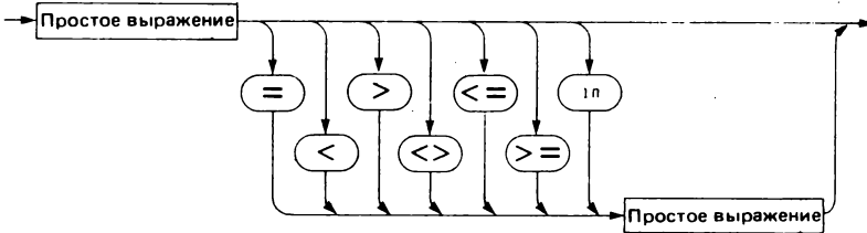
Рис. 4.8. Синтаксическая диаграмма для Выражения
