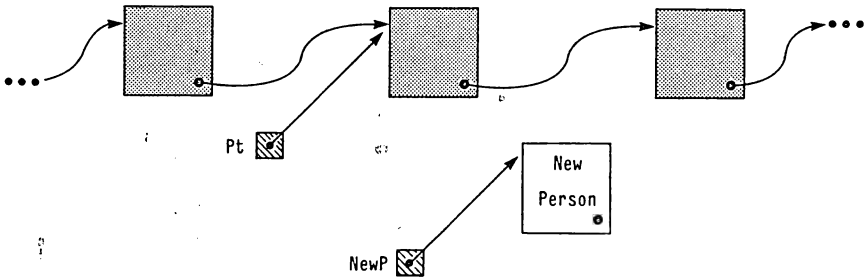
Рис. 10.4. Связный список перед включением
