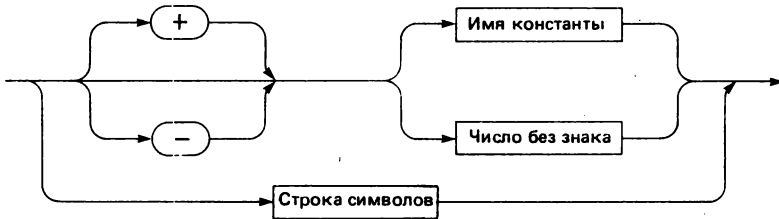
Р и с. 3.7. Синтаксическая диаграмма для Константы
