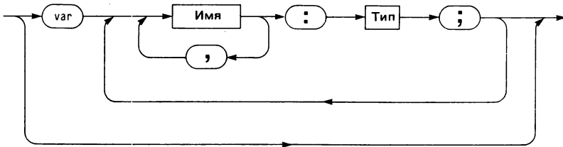
Рис. 3.10. Синтаксическая диаграмма для Раздела описания переменных
