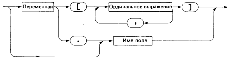
Рис. 6.3. Синтаксическая диаграмма для Переменной-компоненты
