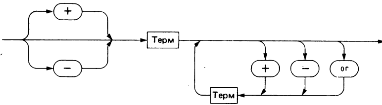
Рис. 4.7. Синтаксическая диаграмма для Простого выражения
