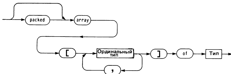
Р и с. 6.4. Синтаксическая диаграмма для Массивового типа
