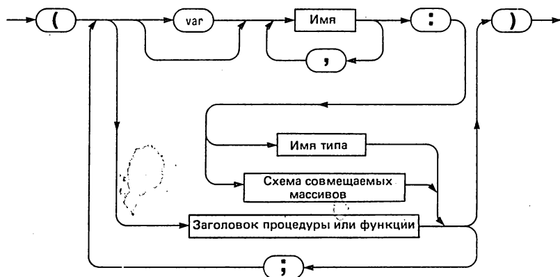
Рис. 11.5. Синтаксическая диаграмма для Списка формальных параметров
