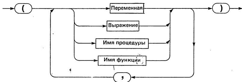
Рис. 11.6. Синтаксическая диаграмма для Списка фактических параметров
