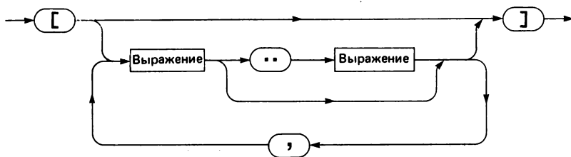
Р и с. 8.2. Синтаксическая диаграмма для Конструктора множества
