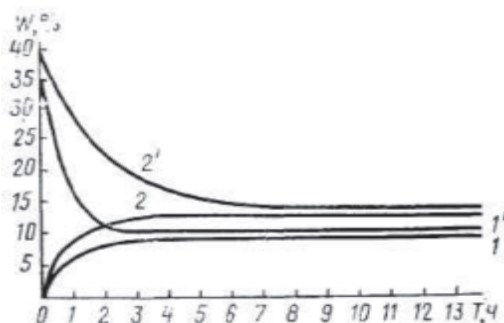
24-rasm. Toʻqimachilik iplari suv bugʻlarining sorbsiyali va desorbsiyali oʻzgarishidagi egri chizigʻi. 1,1ʻ viskoza ipi; 2,2ʻ ipak.
