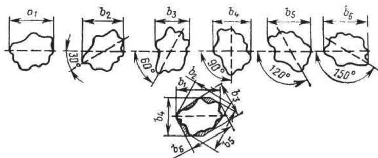
11-rasm. Ipning ko'ndalang kesim yuzasini aylantirish usuli bo'yicha aniqlash.
