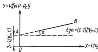
25-rasm. BET doimiy tengligini aniqlash uchun sxema.
