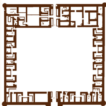
Пайкент. Рабат сызбасы (жоспары). VII ғасыр.
